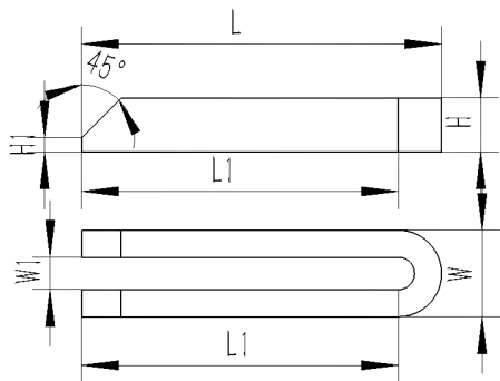
选型示意图
